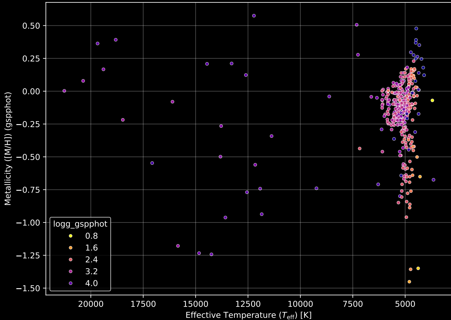
APOGEE DR17 Field: [165+00] Stellar Population Parameters (n= 430)
